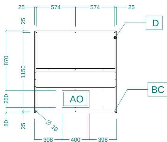
Dessus
